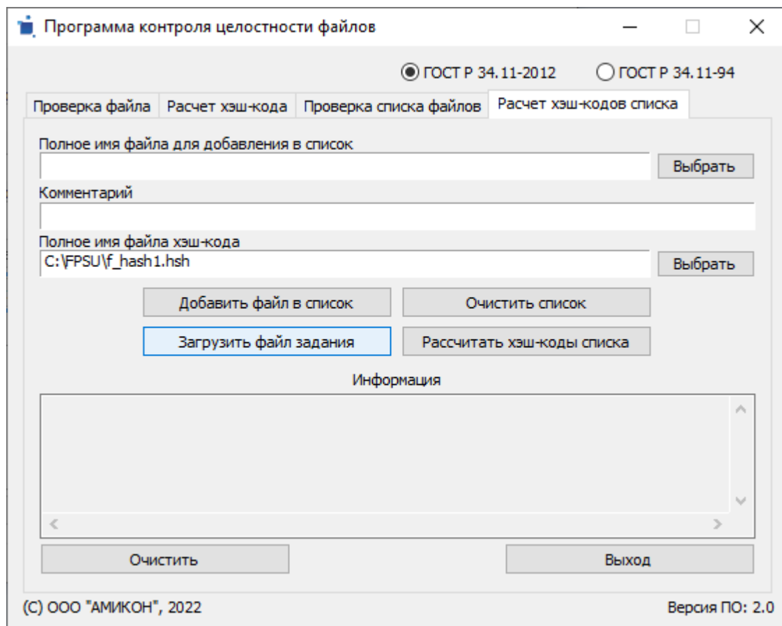
Рисунок 11 - Вкладка «Расчёт хэш-кодов списка»
